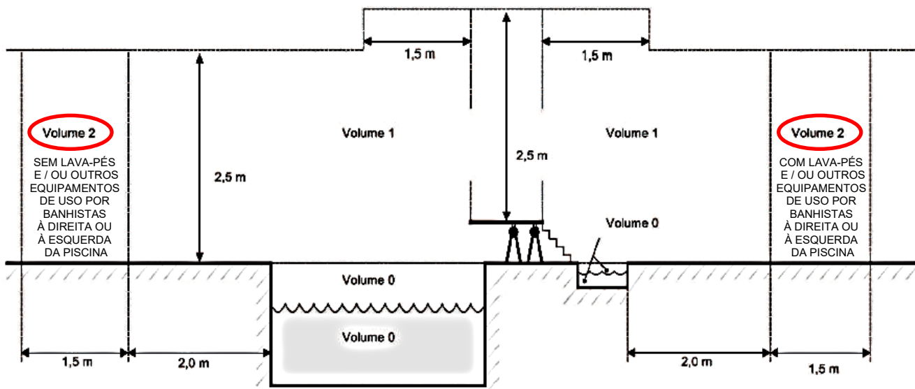
Figura 20 — Dimensões dos volumes para reservatórios de piscinas e lava-pés
