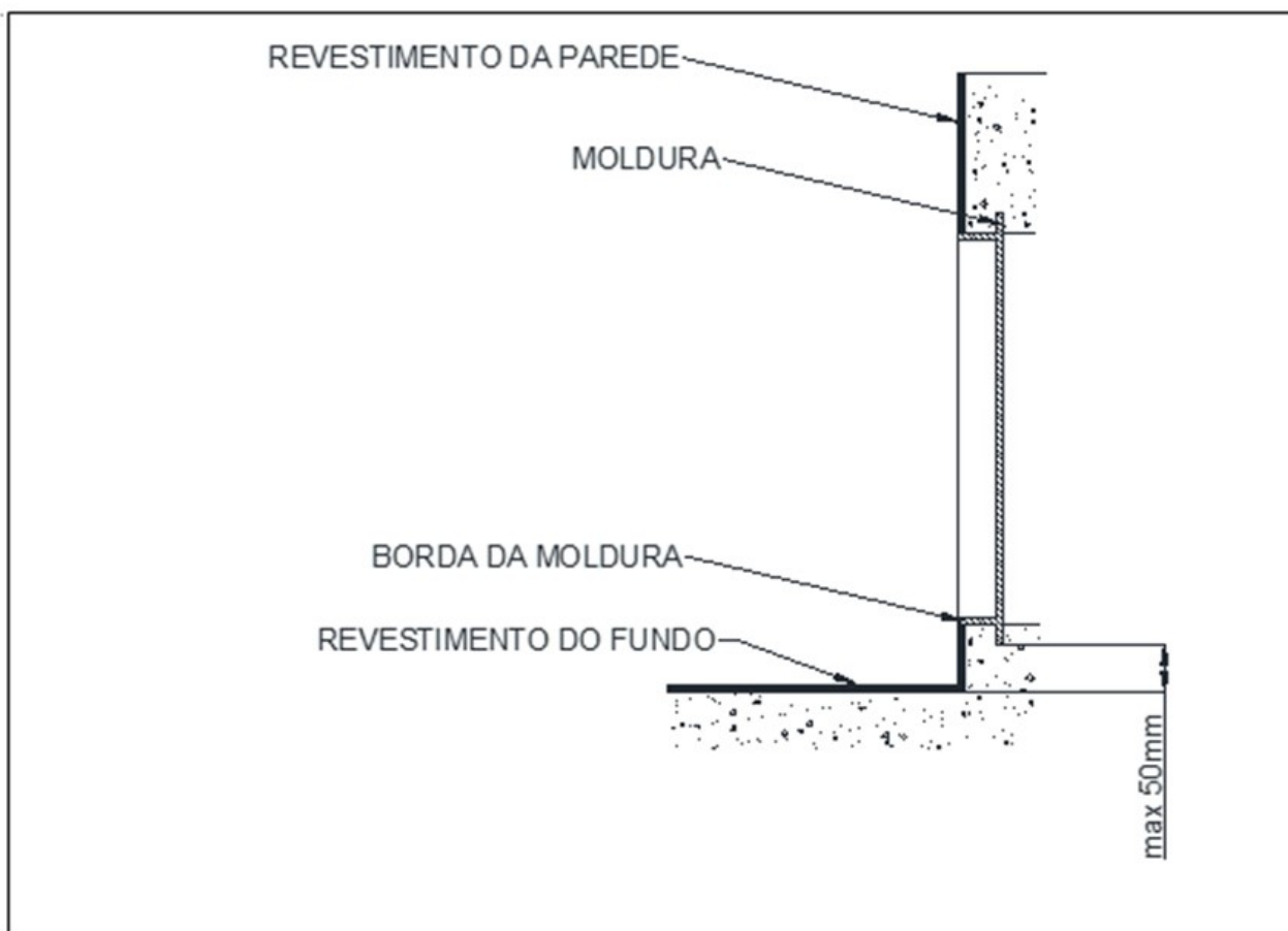
Figura 4 – Parede da Piscina
