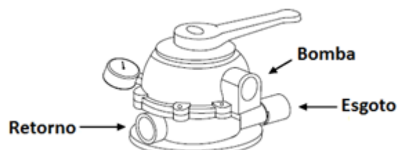
Figura : Válvula Seletora 6 Vias Jacuzzi
